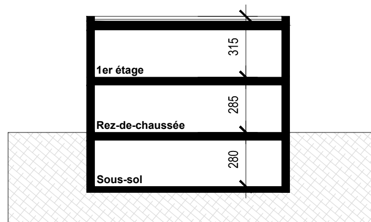
Coupe type - toit plat
