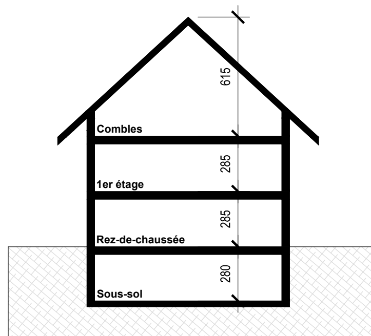
Coupe type - toit en pente
